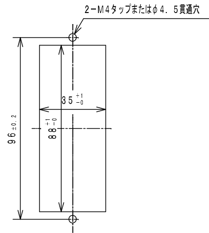
縦形計器パネルカット図
