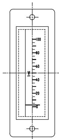
縦形計器正面図
