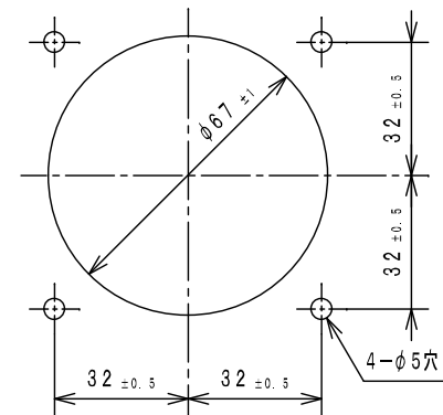
パネルカット図
