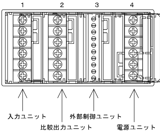
TDR-49TB背面図 端子台番号
