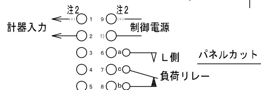
L設定用端子構成及び設定部
