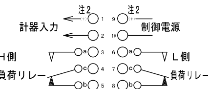
H, L設定用端子構成及び設定部
