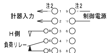
H設定用端子構成及び設定部
