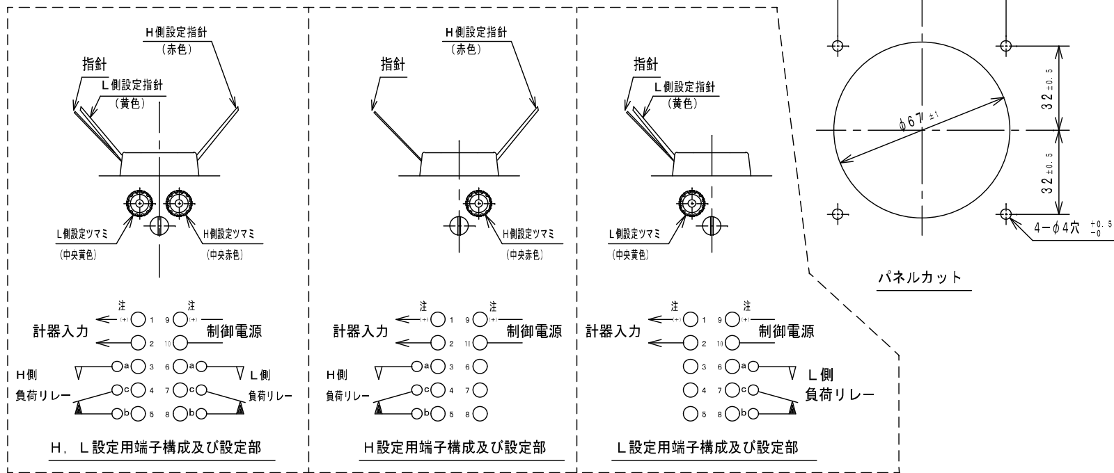
MPC-8 (HL, H, L 設定) 無接点式メータリレー外形図
